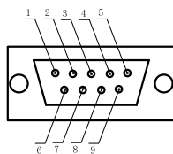
电机接线图
